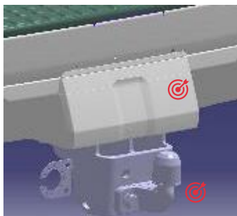
Фланцов теглич с топка PW96060011
